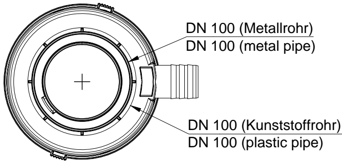
Ansicht von unten from above
